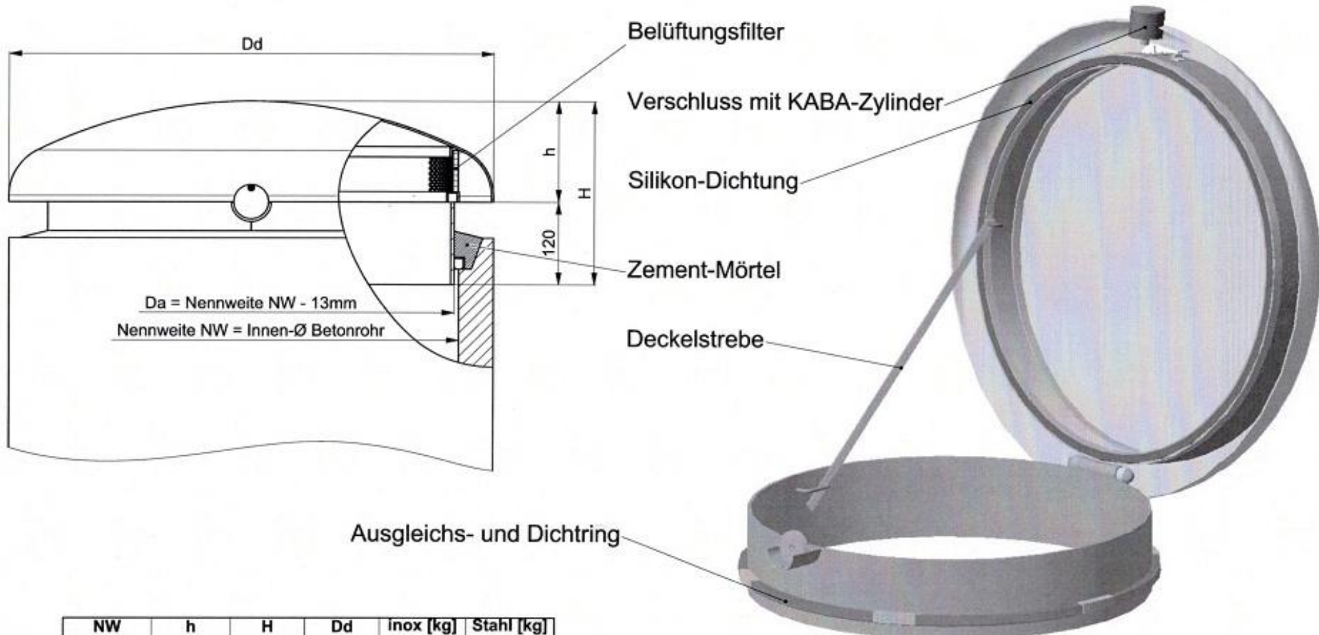
Brunnenstuben- und Reservoirabdeckung mit integrierter Belüftung
