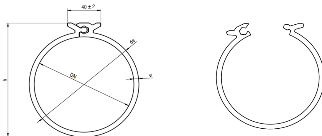
Baulänge 5 m - Längsverschluss Kabelschutzrohre aus LDPE
